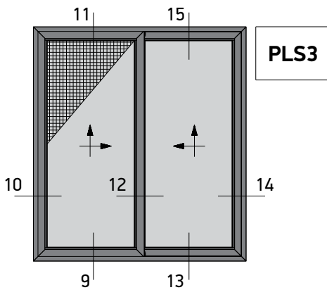
Two Sash Lift and Slide 45° Cut with Flyscreen Right Δίφυλλο Επάλληλο με κοπή 45° και Σήτα Δεξιά Ανάσπυρόμενο
