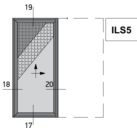
Single Sash Pocket Lift&Slide Window with Narrow Flyscreen and Shutter Μονόφυλλο Χωνευτό Ανασπύρομενο με Στενή Σήτα και Παντζούρι
