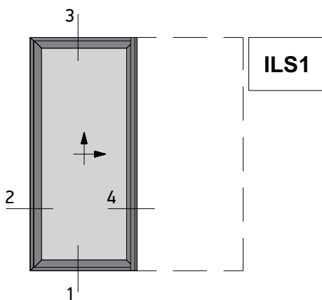
Single Sash Pocket Lift&Slide Window Μονόφυλλο Χωνευτό Ανασπύρομενο
