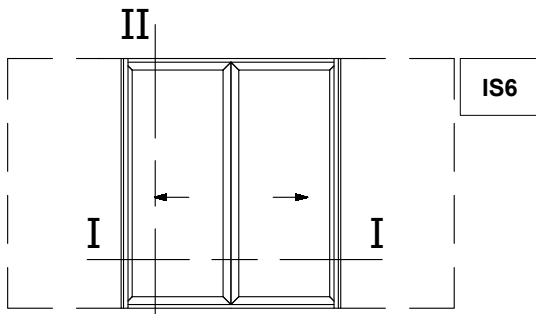
Pocket Sliding Window with Meeting Stile Χωνευτό Συρόμενο Φιλητό
