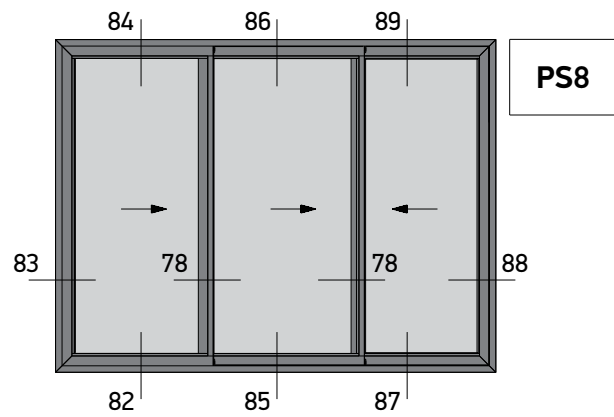
Three Sash Sliding Window 90° Cut (Sash M4544) Right Τρίφυλλο Επάλληλο με κοπή 90° (φύλλο M4544) Δεξιά Συρόμενο
