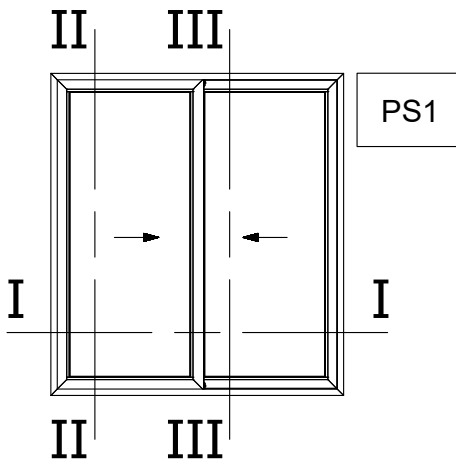
Two Sash Sliding Window 45° Cut Right Δίφυλλο Επάλληλο με κοπή 45° Δεξιά Συρόμενο
