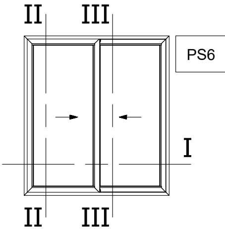
Two Sash Sliding Window 45° Cut (Sash M4542) Right Δίφυλλο Επαλληλο με κοπή 45° (Φύλλο M4542) Δεξιά Συρόμενο
