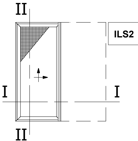
Single Sash Pocket Lift&Slide Window with Flyscreen Μονόφυλλο Χωνευτό Ανασπώμενο με Σήτα
