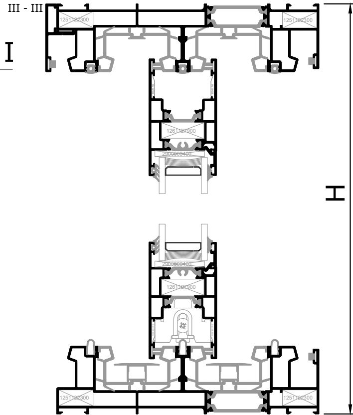
Three Sash Sliding Window 90° Cut (Sash M4544) Right Τρίφυλλο Επάλληλο με κοπή 90° (φύλλο M4544) Δεξιά Συρόμενο
