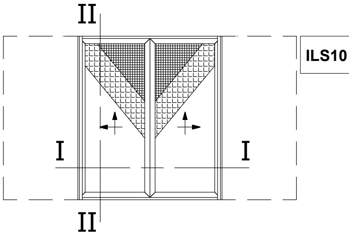
Pocket Lift&Slide Window with Meeting Stile, with Narrow Flyscreen and Shutter Χωνευτό Ανασπυρόμενο Φιλητό με Στενή Σήτα και Παντζούρι
