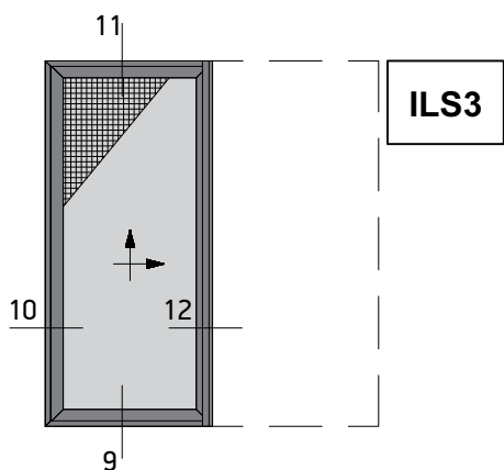
Single Sash Pocket Lift&Slide Window with Narrow Flyscreen Μονόφυλλο Χωνευτό Ανασπύρομενο με Στενή Σήτα
