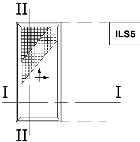
Single Sash Pocket Lift&Slide Window with Narrow Flyscreen and Shutter Μονόφυλλο Χωνευτό Ανασπώμενο με Στενή Σήτα και Παντζούρι
