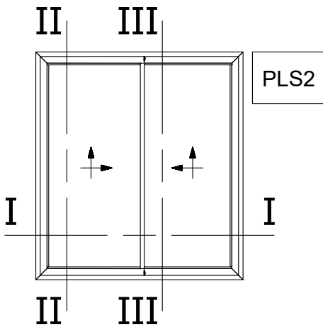
Two Sash Lift and Slide 90° Cut Right Δίφυλλο Επάλληλο με κοπή 90° Δεξιά Ανάσυρόμενο
