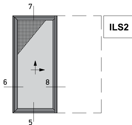
Single Sash Pocket Lift&Slide Window with Flyscreen Μονόφυλλο Χωνευτό Ανασπύρομενο με Σήτα
