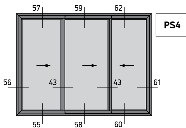
Three Sash Sliding Window 90° Cut Right Τρίφυλλο Επάλληλο με κοπή 90° Δεξιά Συρόμενο
