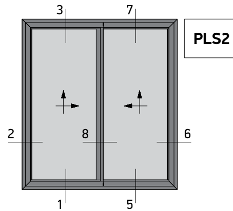
Two Sash Lift and Slide 90° Cut Right Δίφυλλο Επάλληλο με κοπή 90° Δεξιά Ανάσπυρόμενο
