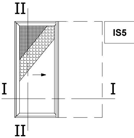
Single Sash Pocket Sliding Window with Narrow Flyscreen and Shutter Μονόφυλλο Χωνευτό Συρόμενο με Στενή Σήτα και Παντζούρι
