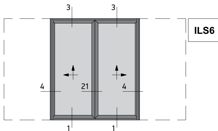
Pocket Lift&Slide Window with Meeting Stile Χωνευτό Ανασπύρομενο Φιλητό
