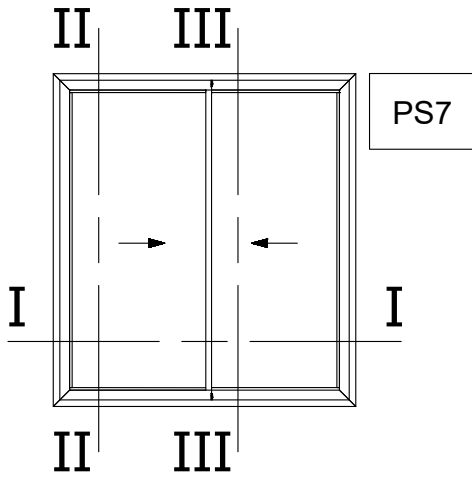
Two Sash Sliding Window 90° Cut (Sash M4544) Right Δίφυλλο Επάλληλο με κοπή 90° (Φύλλο M4544) Δεξιά Συρόμενο
