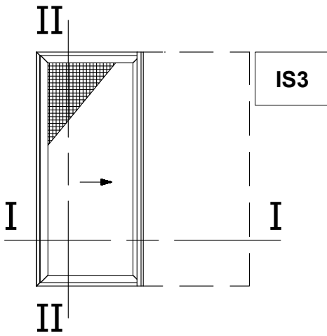
Single Sash Pocket Sliding Window with Narrow Flyscreen Μονόφυλλο Χωνευτό Συρόμενο με Στενή Σήτα
