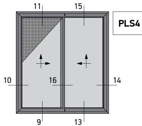
Two Sash Lift and Slide 90° Cut with Flyscreen Right Δίφυλλο Επάλληλο με κοπή 90° και Σήτα Δεξιά Ανάσπυρόμενο
