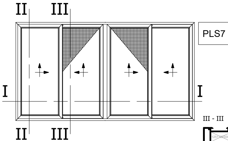
Four Sash Lift and Slide 45° Cut with Flyscreen Right Τετράφυλλο Επάλληλο με κοπή 45° και Σήτα Δεξιά Ανάσυρόμενη
