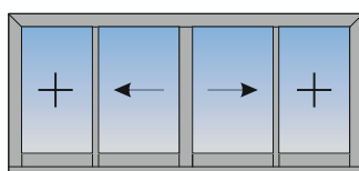
Δίφυλλο επάλληλο συρόμενο με σταθερό
