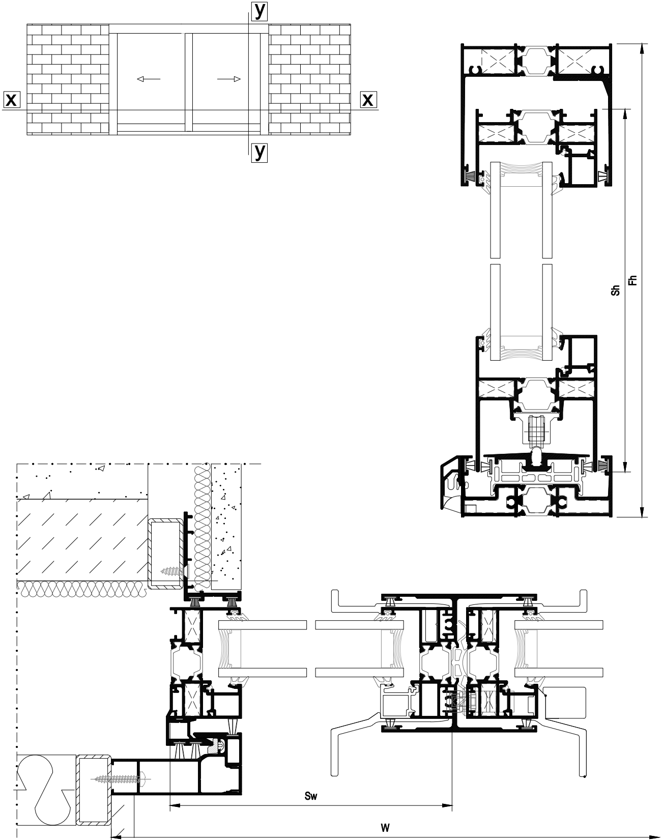
K Δίφυλλο φιλητό χωνευτό Two sash with meeting stile pocket window
